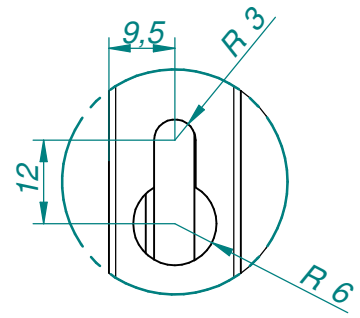
SZCZEGÓŁ B
